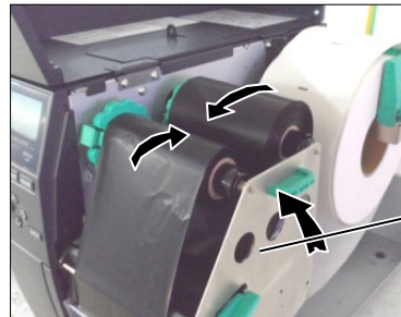
리본 샤프트 홀더 플레이트
