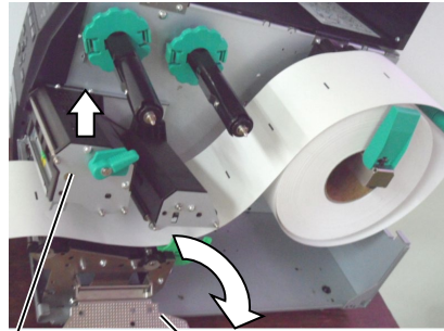
프린트 헤드 뭉치
